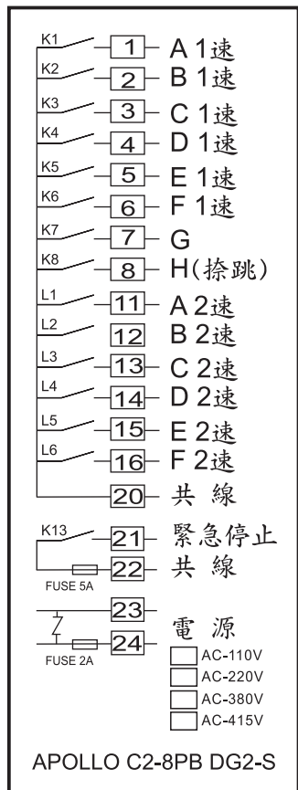
接線圖
